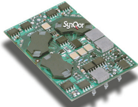
PQ60120QGA08 Module
